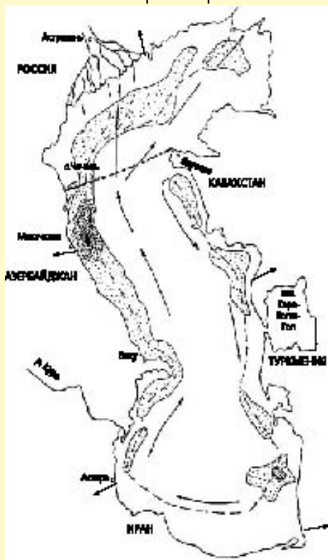
Рис. 1. Распределение осетровых в летний период:
