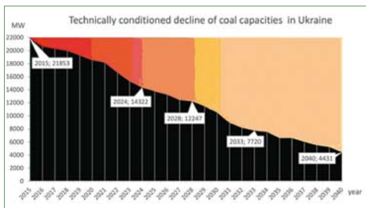
Рис. 6. Технически обусловленное снижение угольных мощностей в Украине
