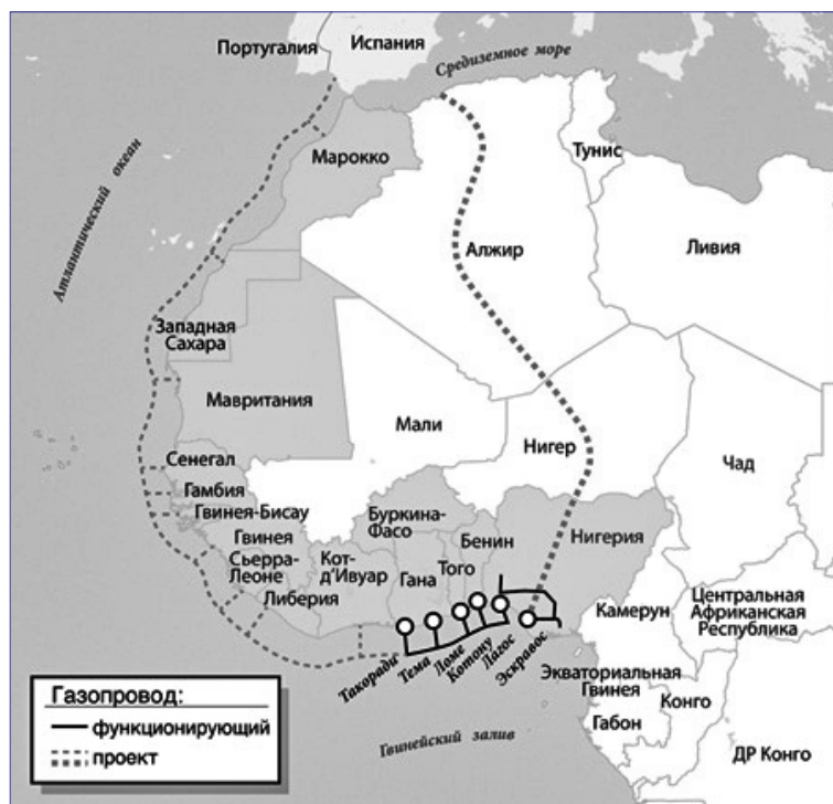
Рис. 7. Проект газопровода Нигерия – Марокко
