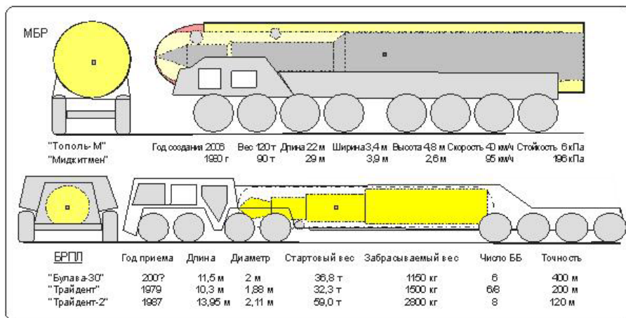
Рис. 3. Российские и американские ракеты: сравнительные данные
